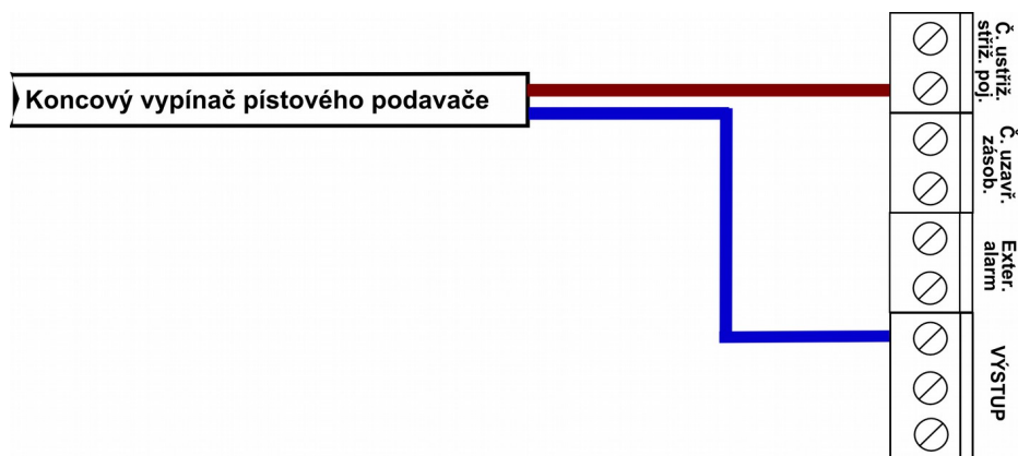
Obrázek 15: Zapojení koncového vypínače pístového podavače
