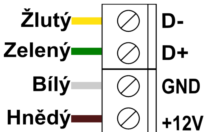
Obrázek 1: Zapojení panelu Standard
