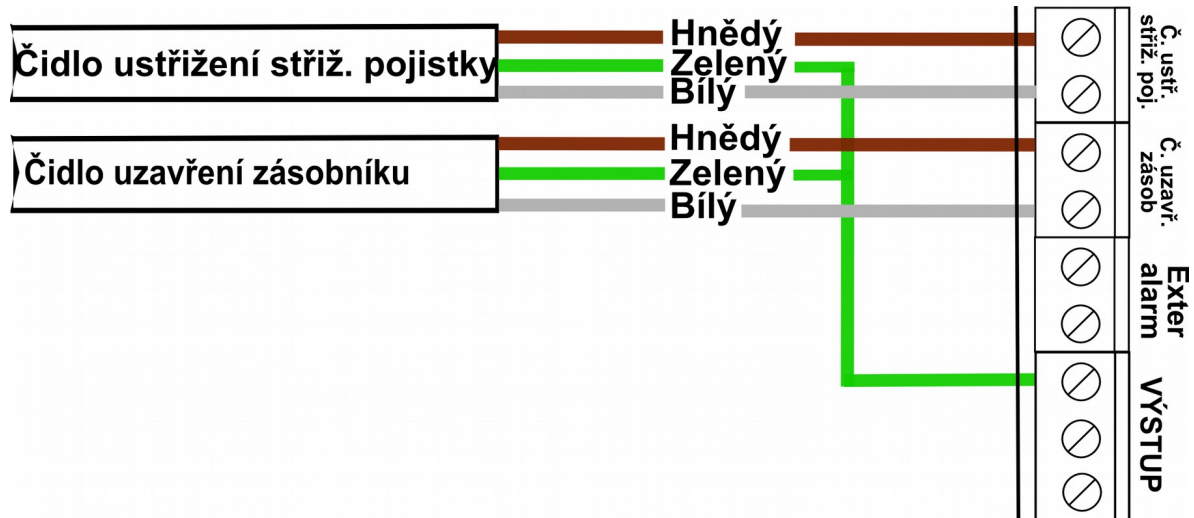
Obrázek 3: Připojení čidel: střížení pojistky podavače (závlačky) a uzavření zásobníku
